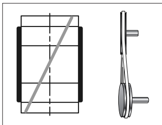
Fig 5 Indicación de desalineación angular vertical
