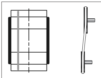
Fig 7 Indicación de desalineación paralela
